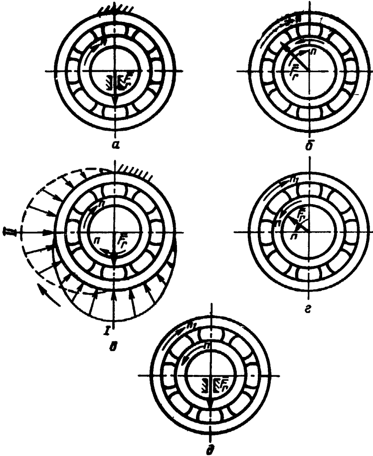
a, б — циркуляционное нагружение внутреннего кольца; в, г — циркуляционное нагружение наружного кольца; д — циркуляционное нагружение обоих колец
